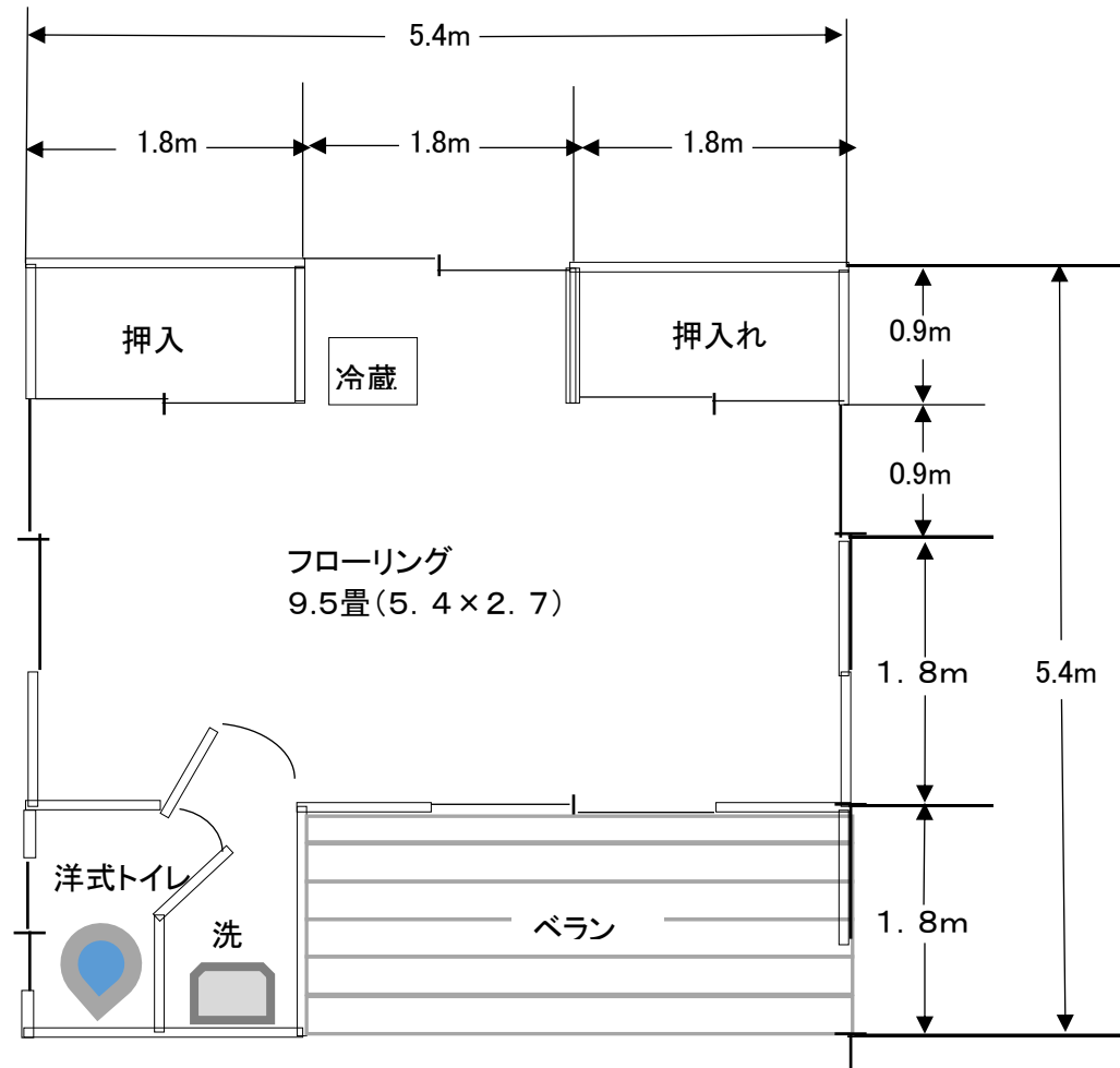
5人棟ログハウス平面図
