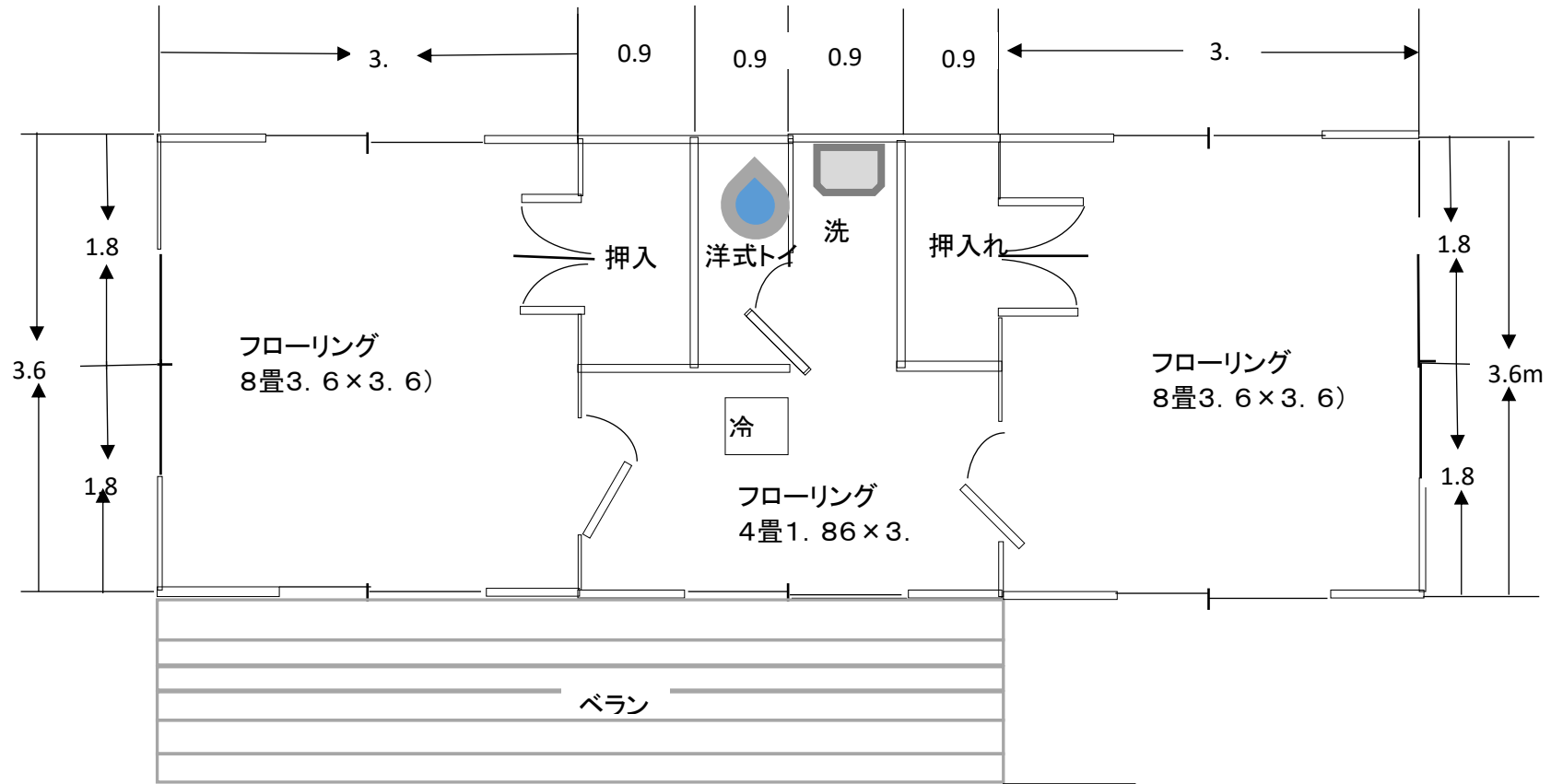
10人棟ログハウス平面図
